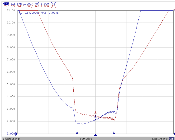
VSWR
